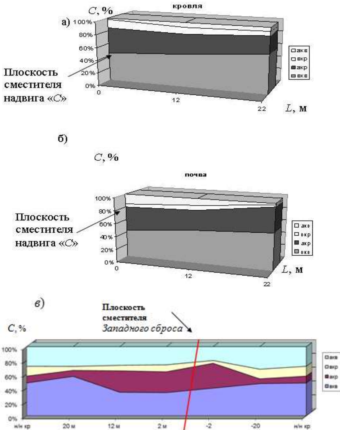
Рисунок 3 – Изменение фазового состояния кварца ( C , %) в породах кровли (а) и почвы (б) пласта m_3 в пределах висячего крыла надвига «С» шахты «Северная» и непосредственной кровли пласта l_1 в зоне влияния Западного сброса шахты «Калиновская - Восточная» (в)
