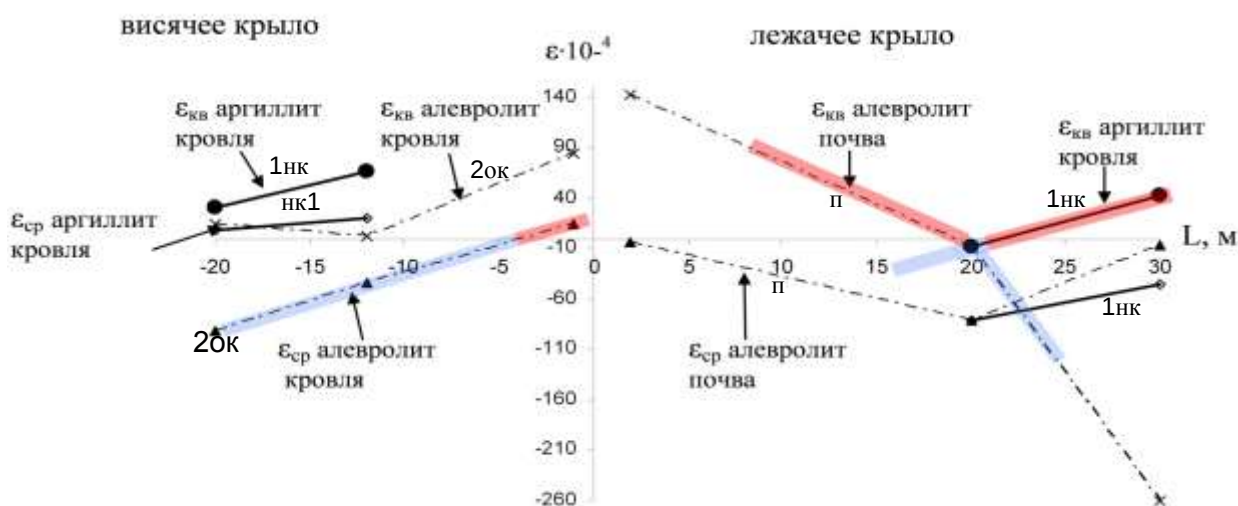
Рисунок 4 – Изменение микродеформаций в породах кровли и почвы пласта l_1 в зоне влияния Западного сброса шахты «Калиновская - Восточная»
